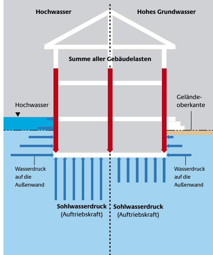
Gefahr des Aufschwimmens: \text{Auftriebskraft} \geq \text{Gebäudelasten}
